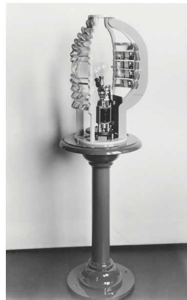
De optiek van Zoutelande, afkomstig uit de oude ijzeren opstand, in proefopstelling bij de Technische Dienst van de Kustverlichting in Scheveningen, vermoedelijk in 1951.
