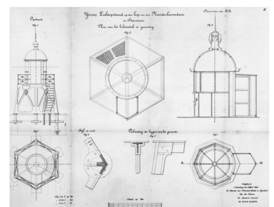
Tekeningen van een ijzeren zeekaap en een lichtopstand voor Stavoren, behorend bij het bestek en voorwaarden van 3 april 1884.
