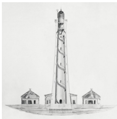
Tekening van de vuurtoren op Schouwen uit 1840. De toren bestaat uit twee cilinders, met daartussen een wenteltrap.
