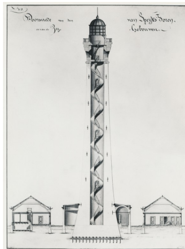
Ontwerp voor de Van-Speijktoren uit 1833. De toren bestaat uit slechts één cilinder.
