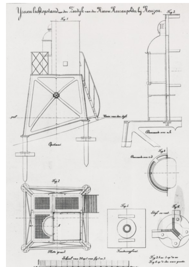
Bestektekening van het lage licht Nieuw-Neuzenpolder uit 1874.
