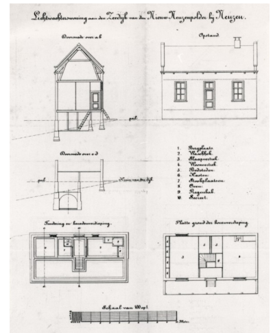
Bestektekening van de lichtwachterswoning Nieuw-Neuzenpolder uit 1874.
