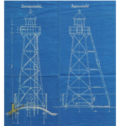
Gedeelte van een blauwdruk van de ontwerptekening van de lichtopstand Den Oever uit 1918.
