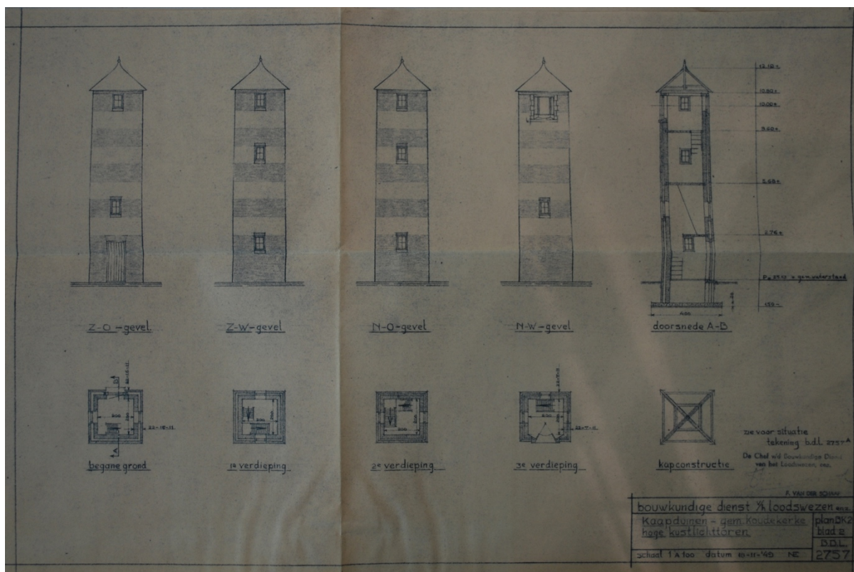
Bouwtekening Hoge Licht Dishoek, 1949, Zeeuws Archief, inv.nr.199
