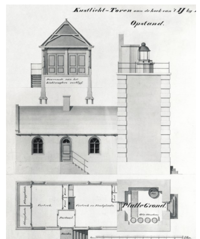
Tekening van de lichtwachterswoning uit 1838.
