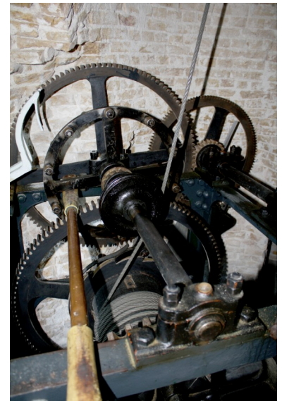
Het uurwerk dat de mistklok laat luiden functioneert nog steeds.
