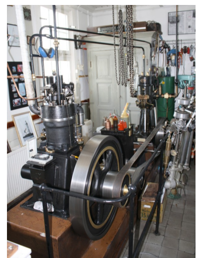
De Bronsmotor voor de productie van perslucht.
