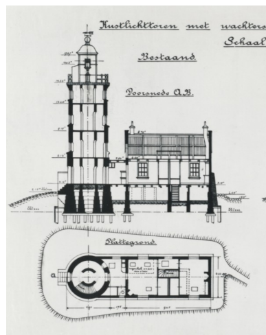
Gedeelte van een revisietekening uit 1918 met daarop de oude situatie, voor de verbouwing.
